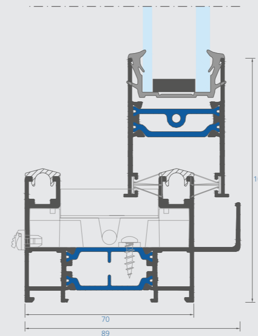
Elégance U w = 1,7
