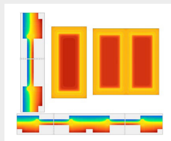
Figura 2 - Termografia de uma janela.
