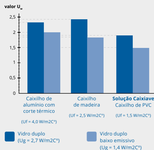
Figura 3 - Transmissão térmica total de várias soluções alternativas de janelas (valor U_w ) para a dimensão de 1m x 1m.
